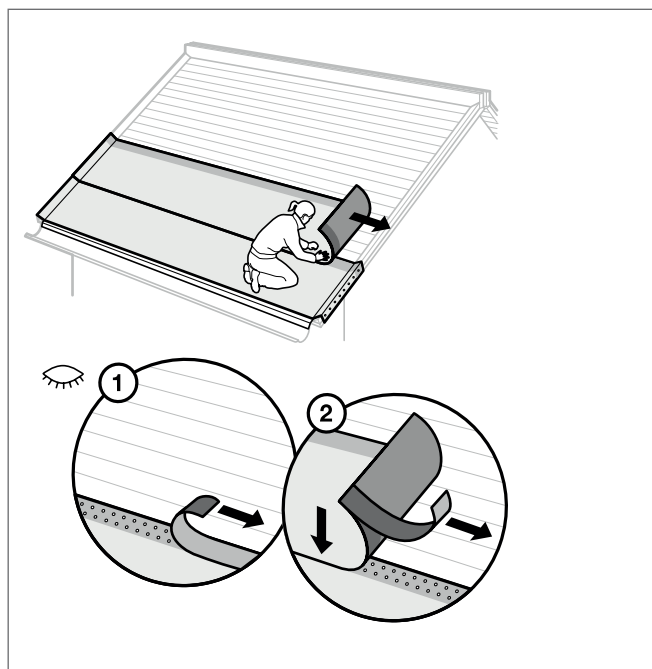
Följande våder
