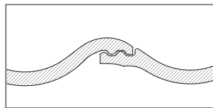
Korrekt sidoförskjutning av pannor
