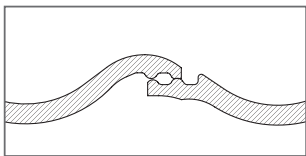
Felaktig sidoförskjutning av pannor.
