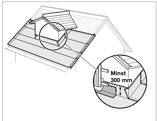
Vertikala uppdragningar.
