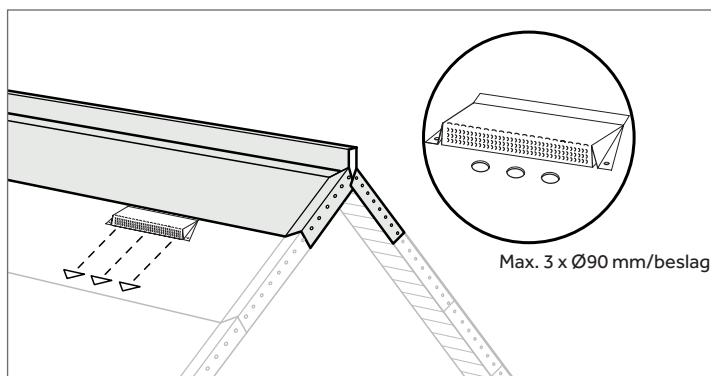
Ventilerad taknock.
